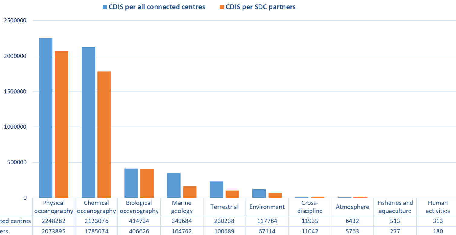
CDIs per SeaDataNet Parameter Disciplines (P08)
